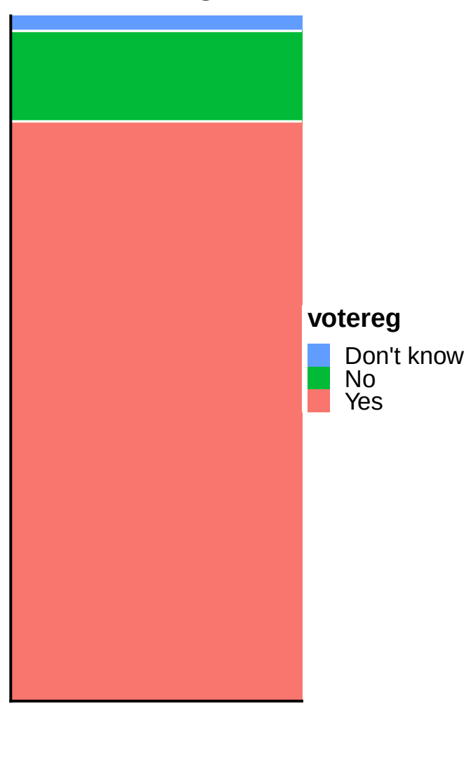
votereg
