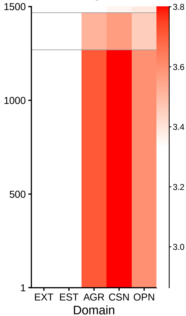
Big5
